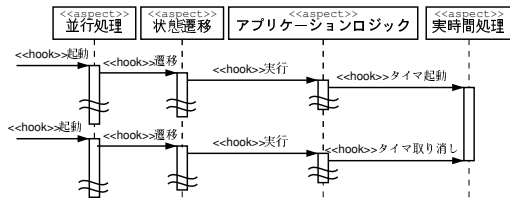
図 4 E-AOSAS+ のシーケンス図
